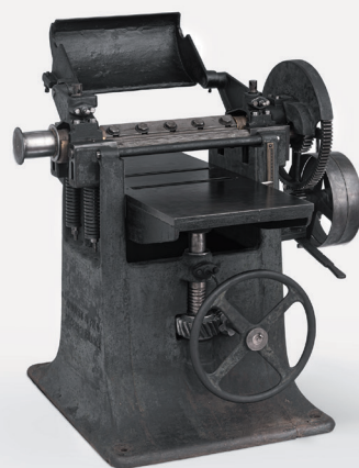
Lodieran arrabotatzeko makina Regruesadora Guilliet & Fils Auxerre, Francia, C.1920
